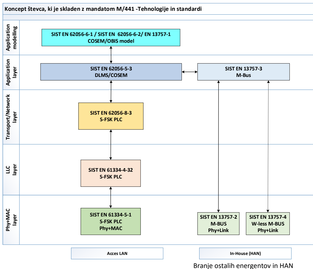
Slika 1: Koncept zahtevanih števcjev v skladu z M/441
